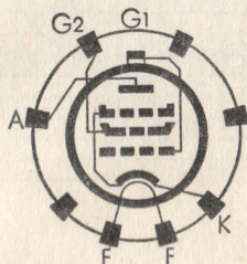
Sockelschaltung
