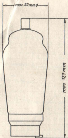
Kolbengröße
